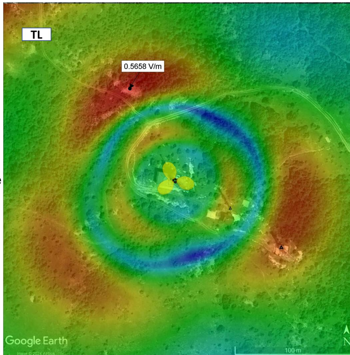
Слика 4.3. Јачина електричног поља на тлу када радио-систем LTE800 оператора Telekom Srbija ради максималним капацитетом
