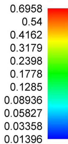
Слика 4.5. Јачина електричног поља на тлу када радио-систем LTE2100 оператора Telekom Srbija ради максималним капацитетом
