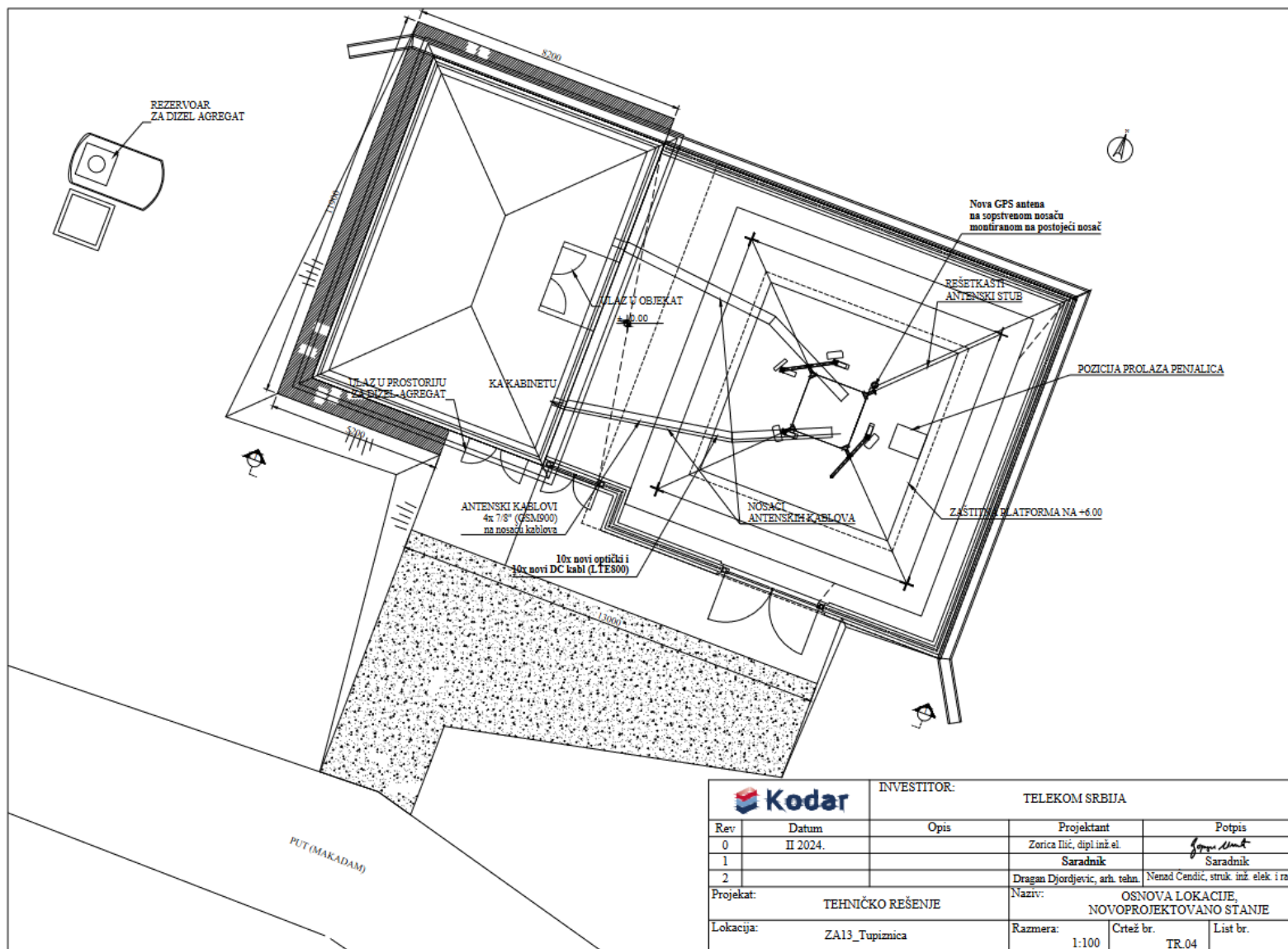
Слика 8.1. Диспозиција опреме на локацији – основа локације – новопроектовано стање
