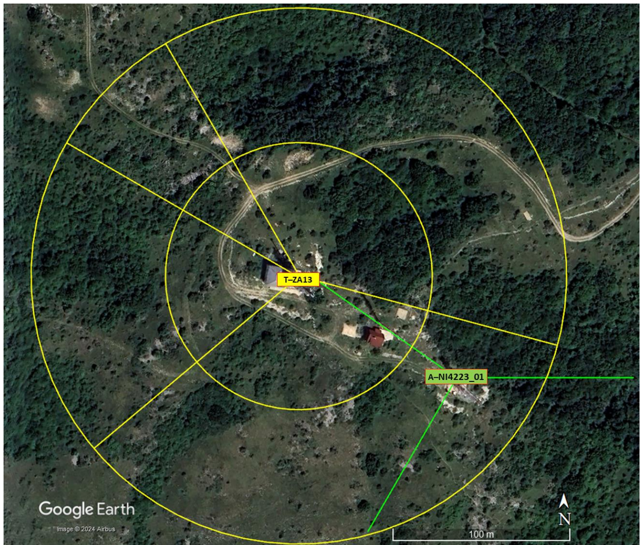
Слика 3.3. Сектори зрачења антена свих извора на локацији
