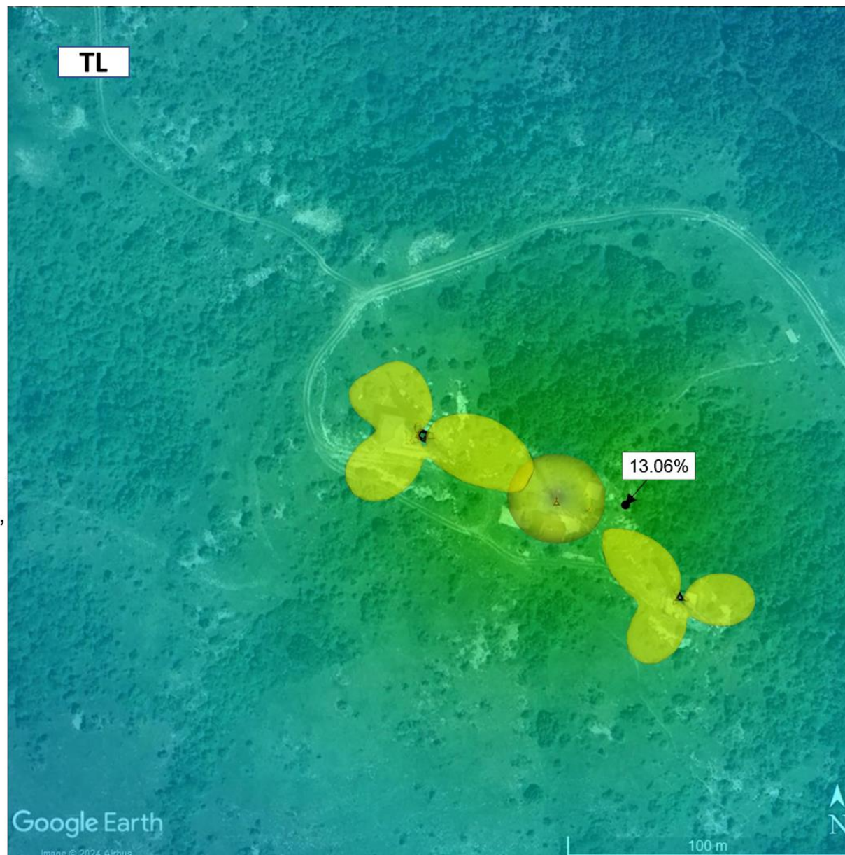
Слика 4.7. Фактор изложености на тлу када сви радио-системи свих оператора на локацији раде максималним капацитетом
